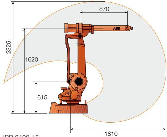
IRB 2400-10, IRB 2400-16
